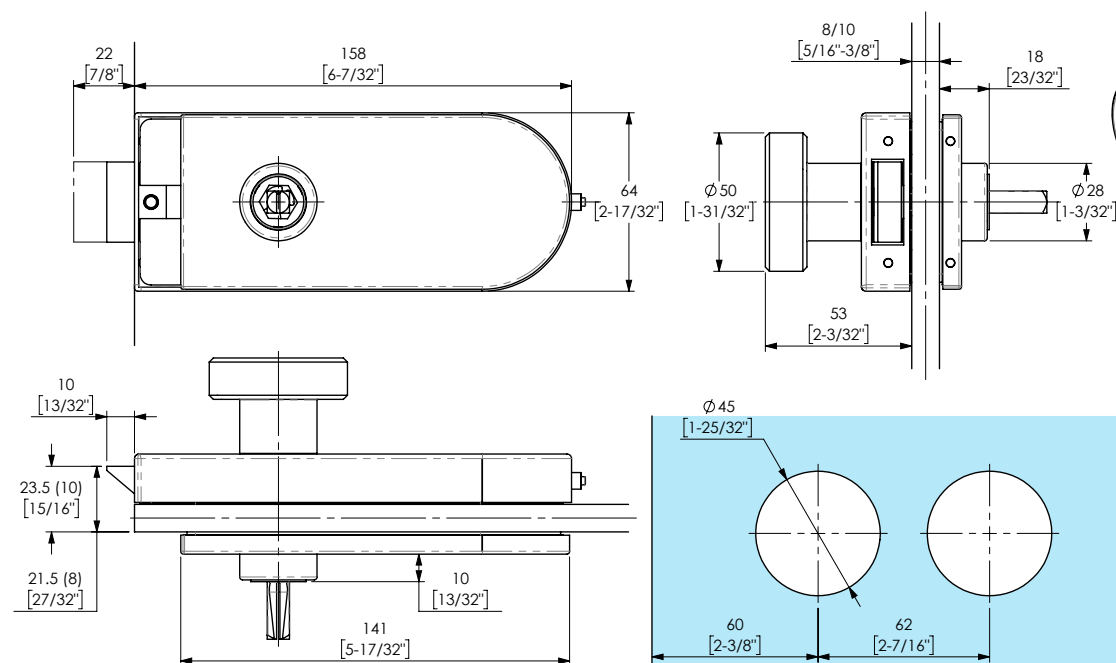
Serratura orizzontale Horizontal lock Cerradura horizontal
